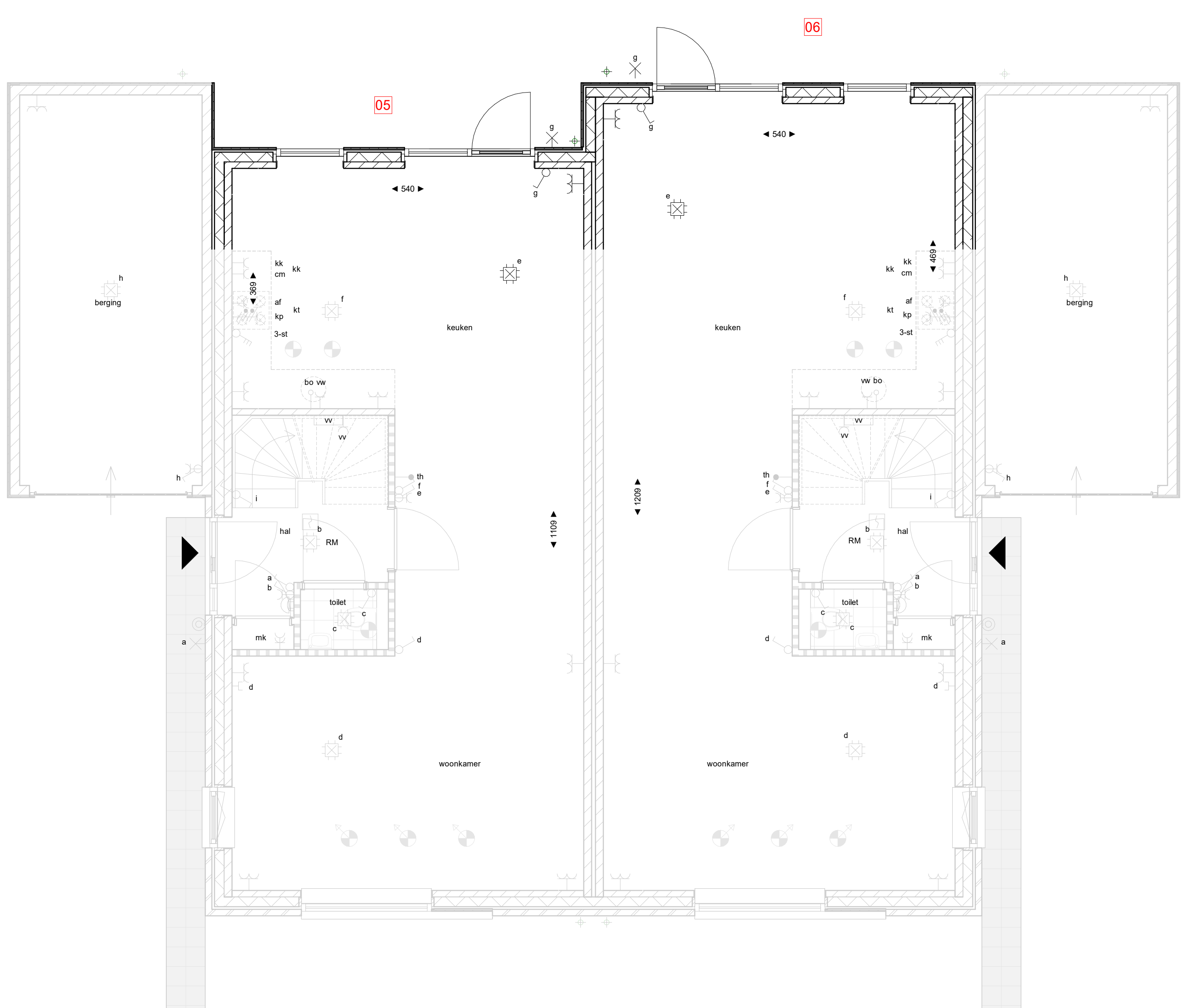
linkergevel 1 : 100
