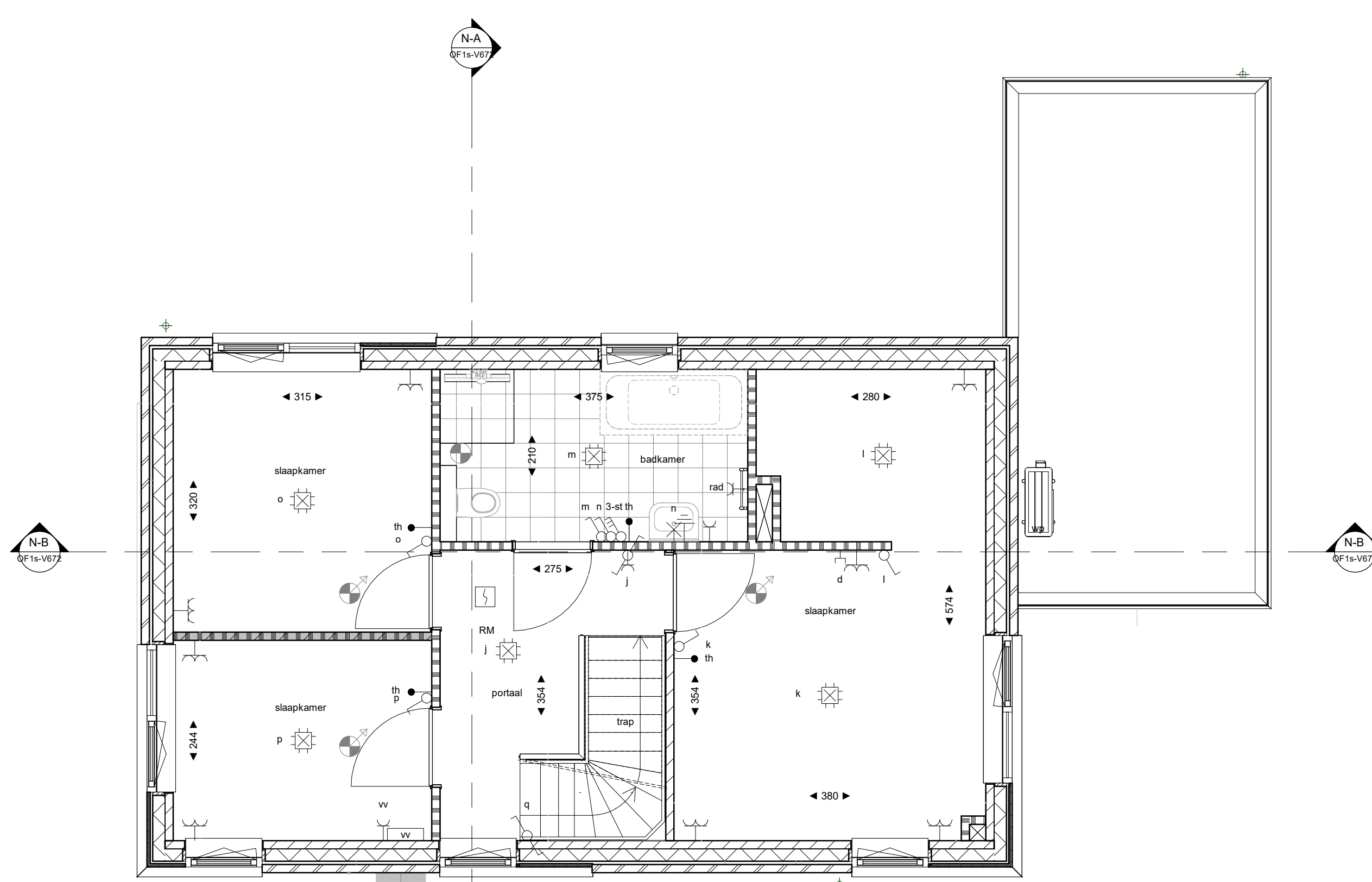
Eerste verdieping 1 : 50
